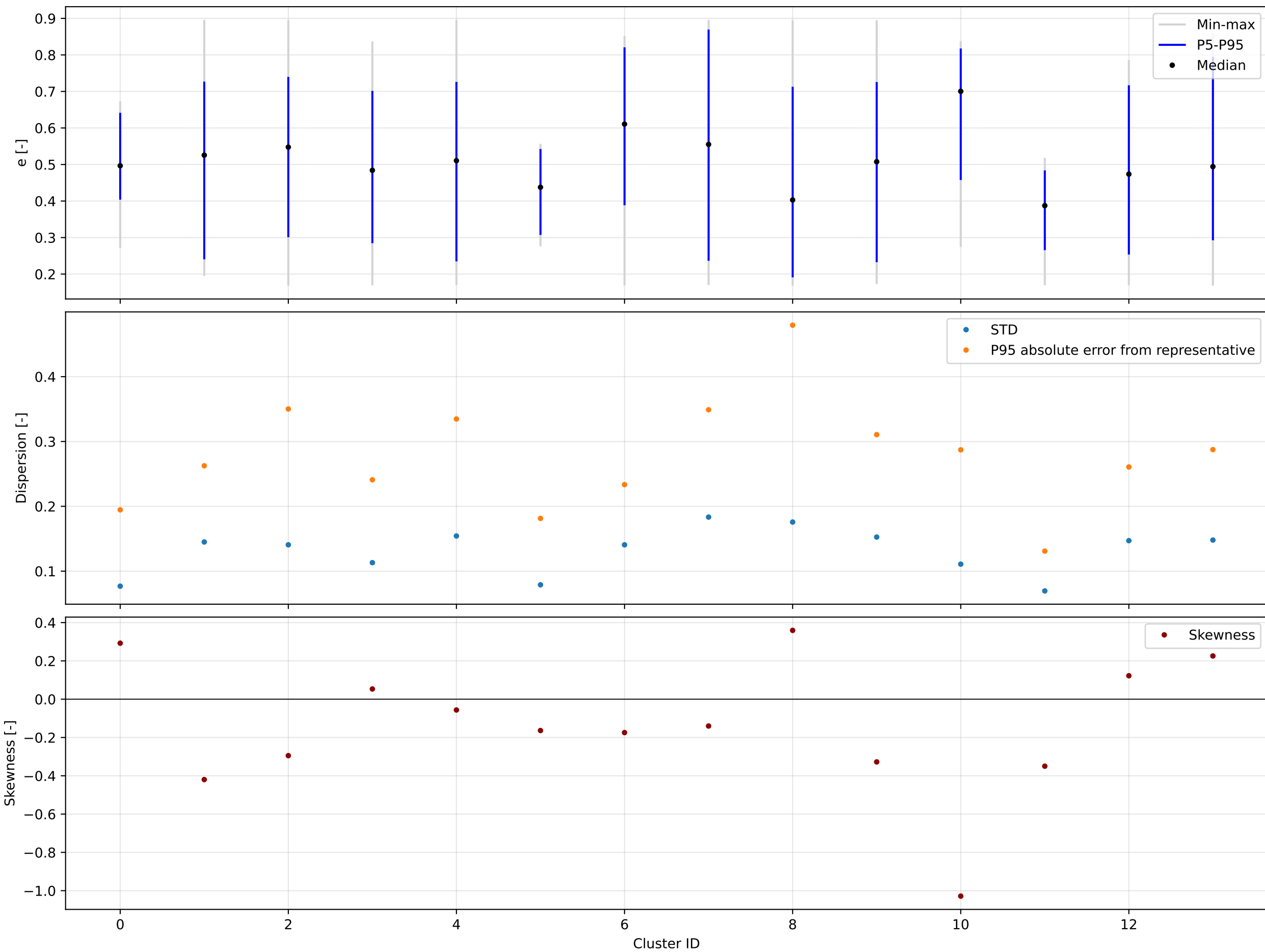
K=14 | backward | e | valid=194058/194058
